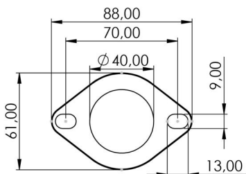
s.s. Flange 38C P/N 207104
